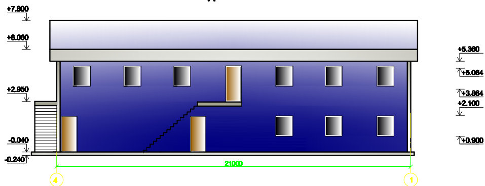
Фасад в осях 4-1
