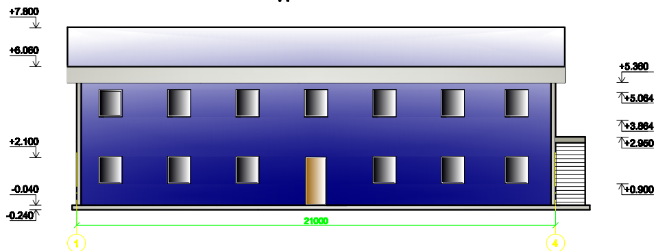
Фасад в осях 1-4
